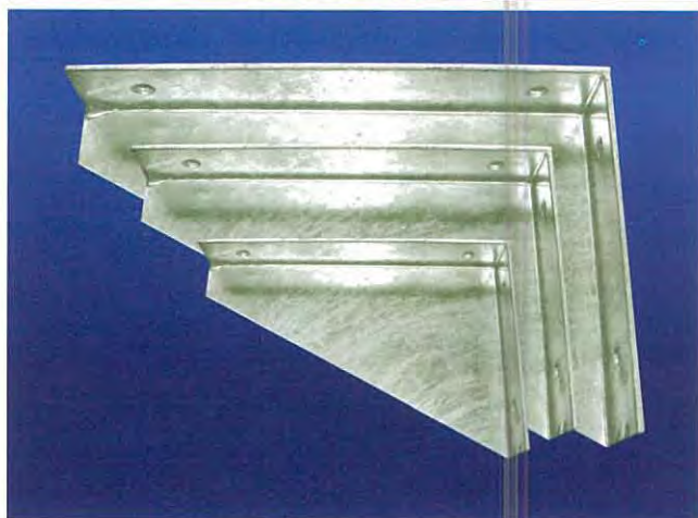
แป้นรองรับเคเบิลแลดเดอร์ - DQRB Bracket Support
